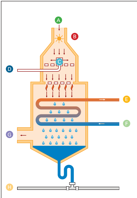
Schema eines Brennwertgerätes Diagram of a condensing appliance
